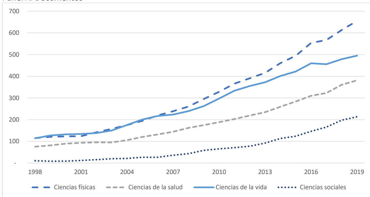
Figura 3. Producción científica a lo largo del tiempo por grandes áreas
